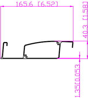
Blade
